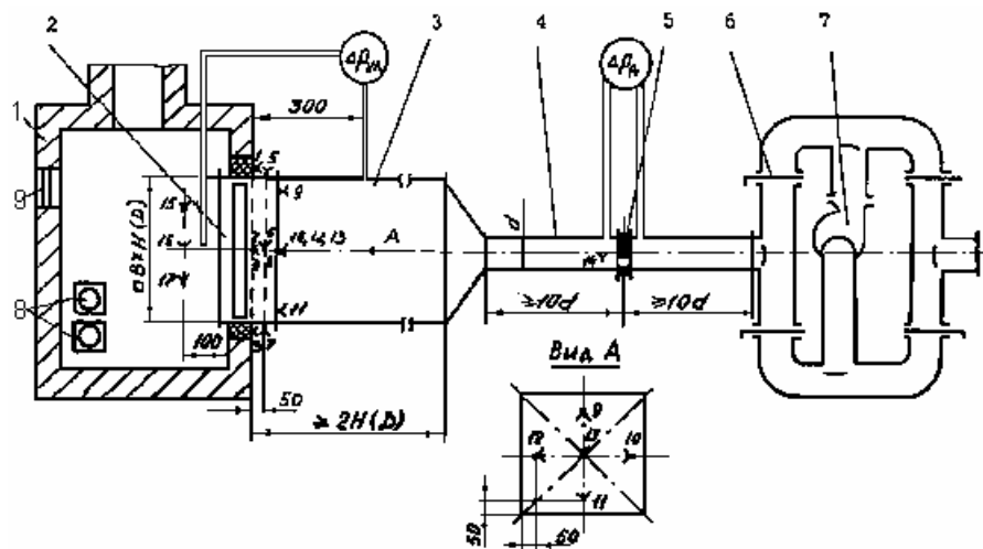
Рис. Б. Схема стендового оборудования для испытаний на огнестойкость огнезадерживающих клапанов для защиты технологических проемов: 1 - печь; 2 - клапан; 3 - воздуховод; 4 - мерный участок воздуховода; 5 - сегментная диафрагма; 6 - регулирующая заслонка; 7 - вентилятор; 8 - форсунки; 9 - иллюминатор; 1-8 - ТЭП диаметром 0,5-0,7 мм, установленные на поверхностях уплотнений корпуса клапана в проеме печи и на поверхностях корпуса клапана; 9-14 - ТЭП диаметром 0,5-0,7 мм, установленные в сечении корпуса клапана и у диафрагмы; 15-17 - ТЭП диаметром 1,2-3,0 мм, установленные в печи; \Delta P_{кл} - перепад давления на клапане; \Delta P_{\delta} - перепад давления на диафрагме
