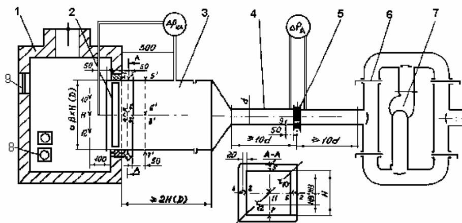
Рис. А. Схема стендового оборудования для испытаний на огнестойкость огнезадерживающих клапанов вентиляционных систем различного назначения:
