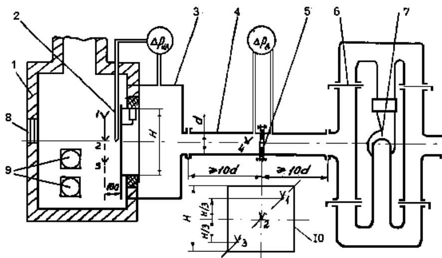
Рис. В. Схема стендового оборудования для испытаний на огнестойкость дымовых клапанов: 1 - печь; 2 - клапан; 3 - переходник; 4 - мерный участок воздуховода; 5 - диафрагма; 6 - регулирующая заслонка; 7 - вентилятор; 8 - иллюминатор; 9 - форсунки; 10 - схема расположения ТЭП в печи относительно клапана:
